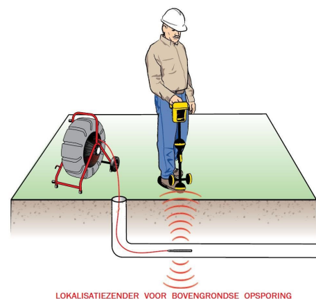
LOKALISATIEZENDER VOOR BOVENGRONDSE OPSPORING
